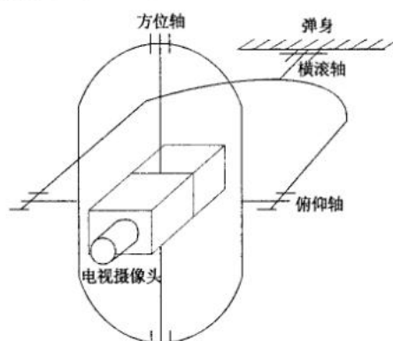
图1 三轴稳定平台的结构示意图
