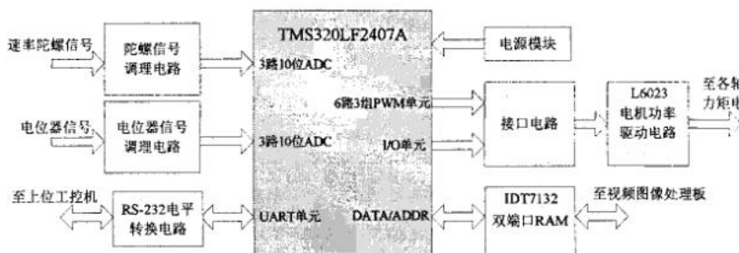
图3 伺服控制板硬件组成框图
