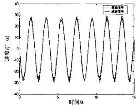
图4 陀螺信号滤波图
