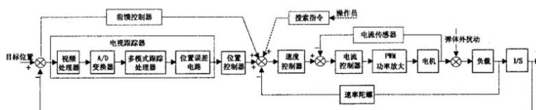
图2 方位轴控制系统结构图
