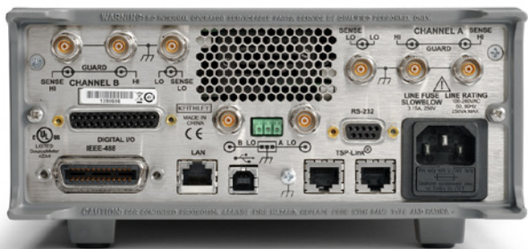
2636B型仪表的背板
