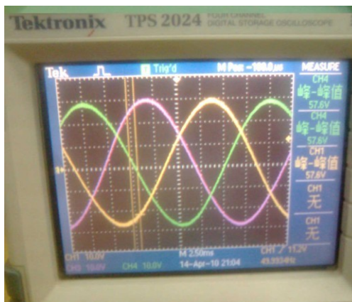
图片 4-1 独立工作模式时纯电阻负载两端的电压波形
