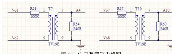
图 3.5 电压互感器电路图
