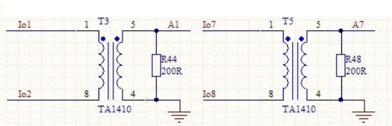
图 3.6 电流互感器电路图
