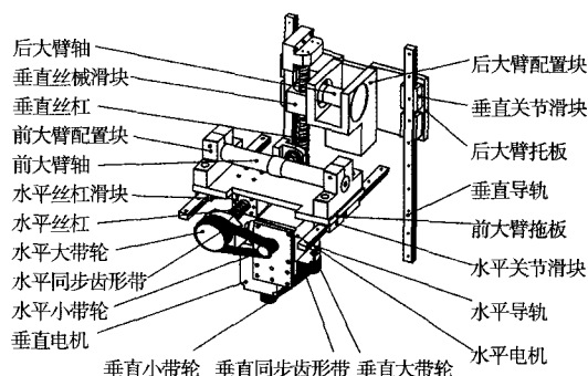
图 2 水平、垂直关节机械构图
