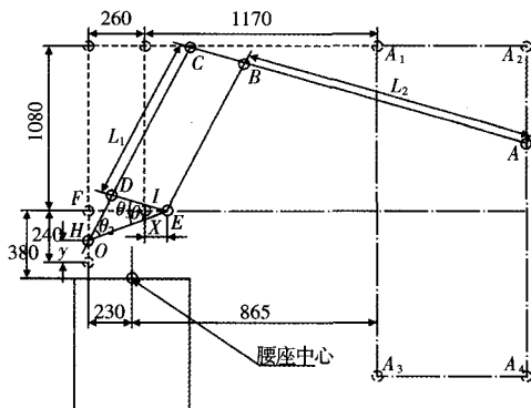
图5 最大工作空间示意图
