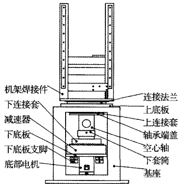
图3 腰部底座关节机械结构图
