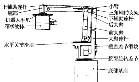
图 1 总体机械结构图
