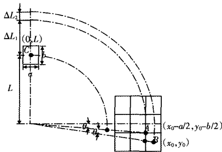
图6 腰部、腕部旋转角度计算简图
