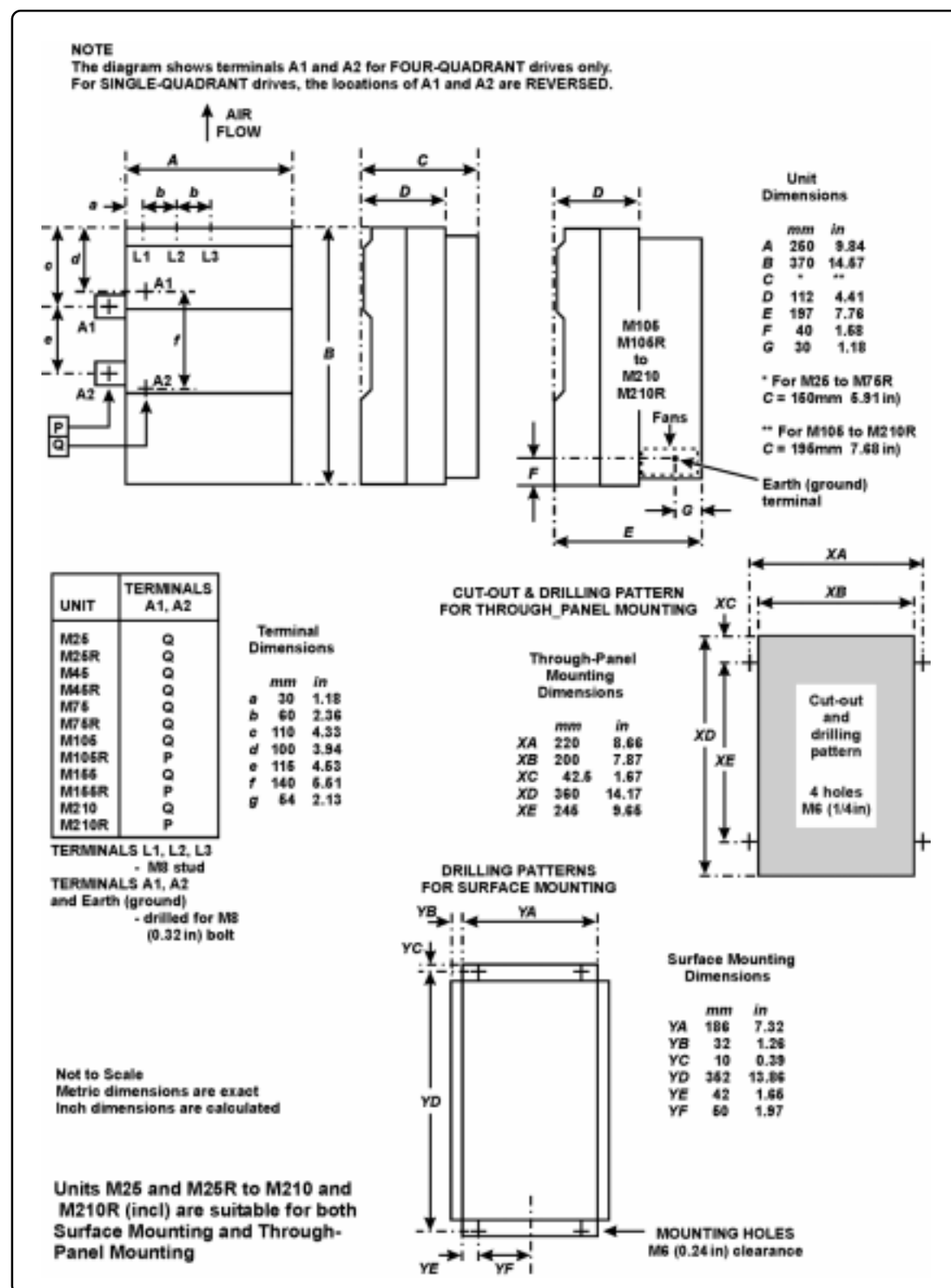
图 8 M25(R)-M210(R)驱动器尺寸及安装方式
