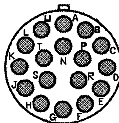
军规接头
